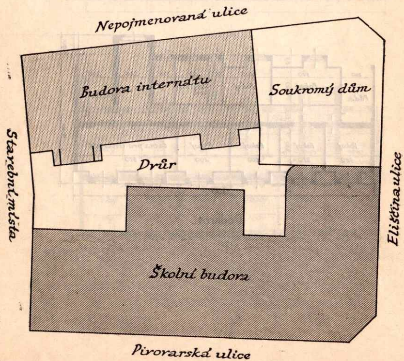
Situační plán 2:400
